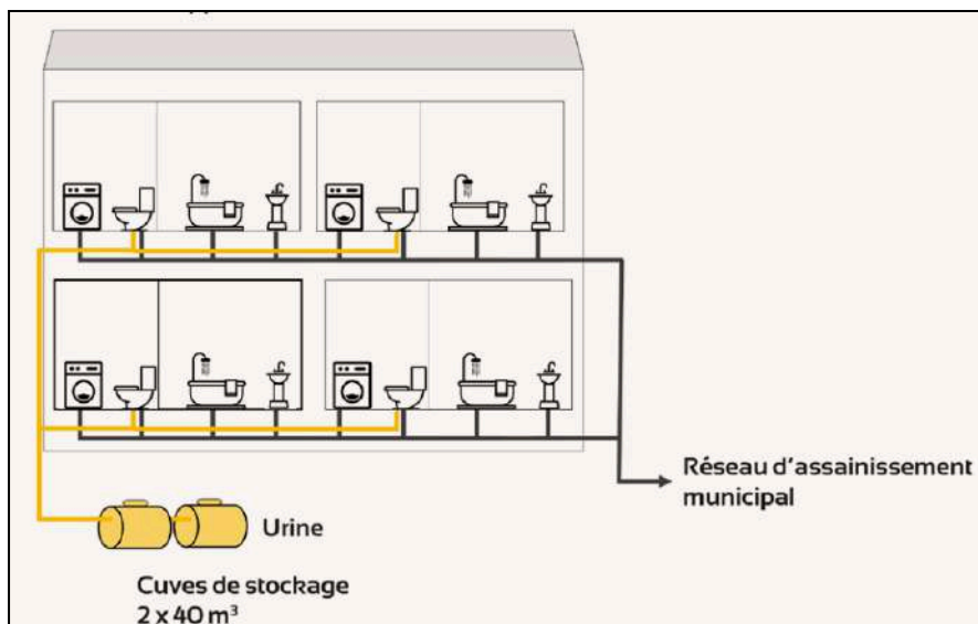
FIGURE 7. Schéma de principe envisageable en zone d'AC. Source : Groupe de travail ARCEAU-IF, Brochure “Quel intérêt pour la séparation à la source dans la gestion des eaux usées domestiques en France ?” , 2021. Schéma de M. Legrand d'après Kim Gutekuns
